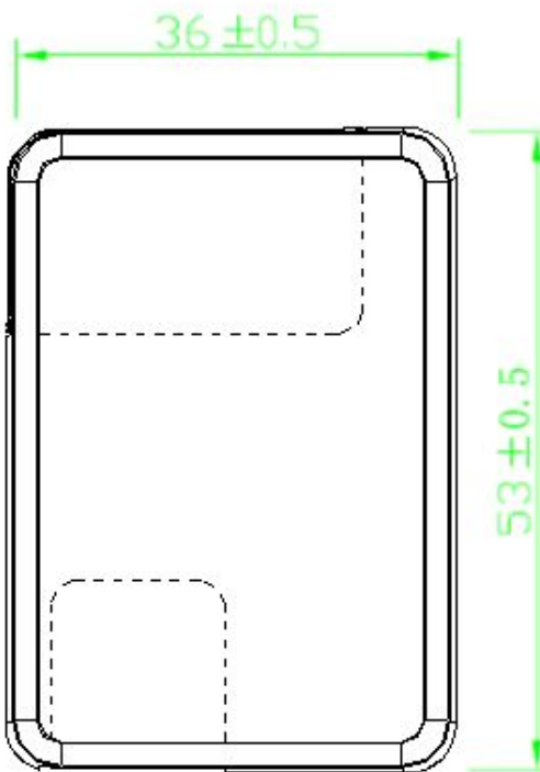
主视图
