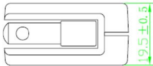
俯视图
